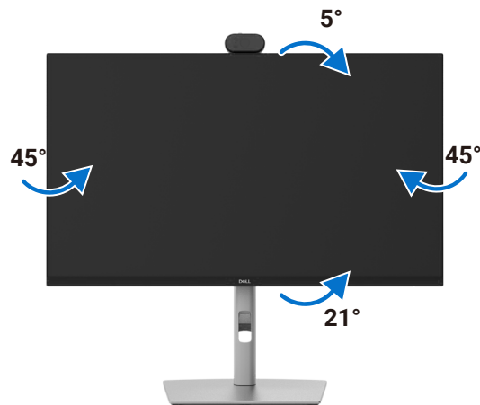
Рисунок 25. Регулировка наклона и поворота (P2426HEV/P2726DEV).
