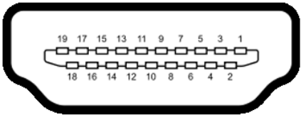
Рисунок 7. Порт HDMI
