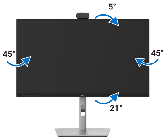
Рисунок 25. Регулировка наклона и поворота (P2426HEB/P2726DEB).
