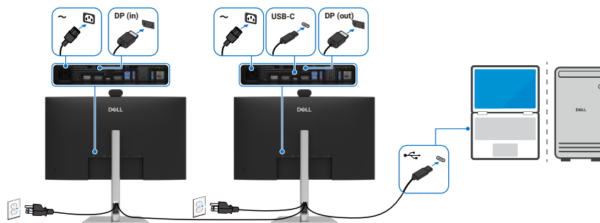
Рисунок 36. Подключение монитора для функции многопоточной передачи (MST)
